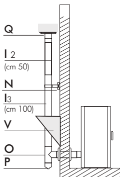
SCHEMA D'INSTALLAZIONE BASE
