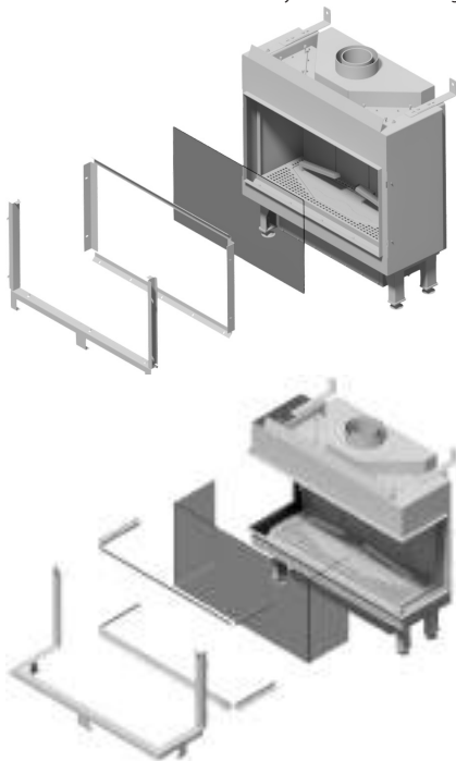
Rys. 18. Sposób demontażu szyby
