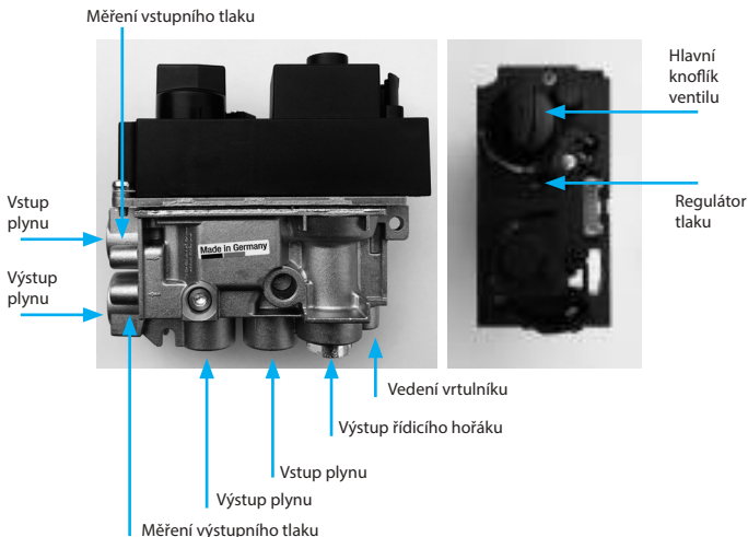
Obr. 20. Regulětor GV60 ve svě zěkladně poloze
